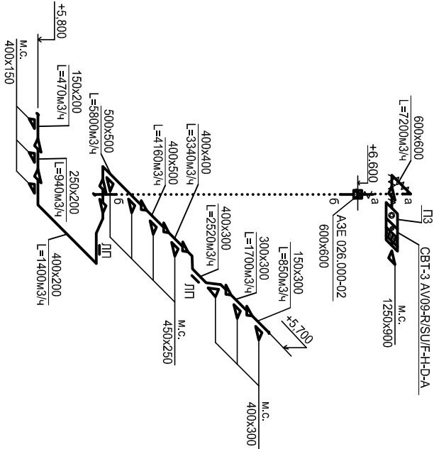
Схема системи П3
